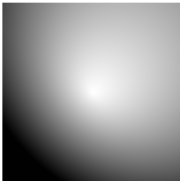
RadialGradient()
